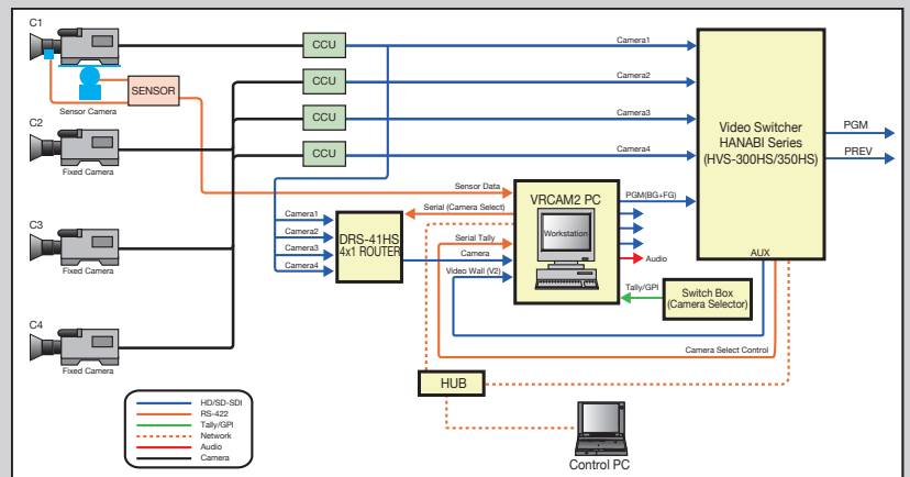
VRCAM2システム例：システムについては弊社スタッフまたは販売代理店までお問合せください。
