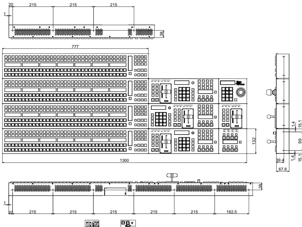
AUX バスユニット
